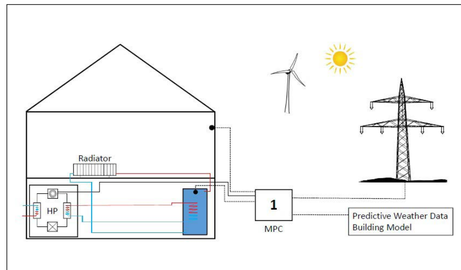
Schéma du câblage et du flux d'information du système de contrôle (MPC) dans le projet Pth4GR 2 ID
